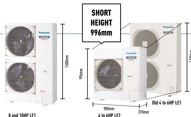
8 and 10HP LE1
